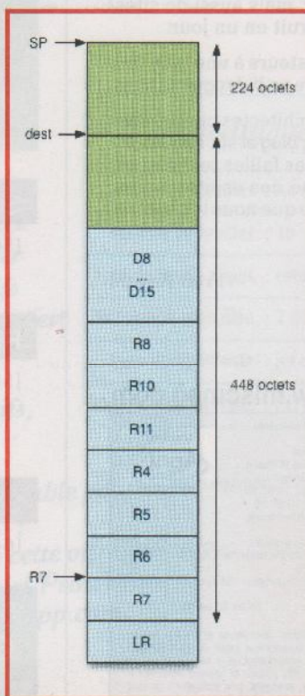
Figure 1 : Etat de la pile
