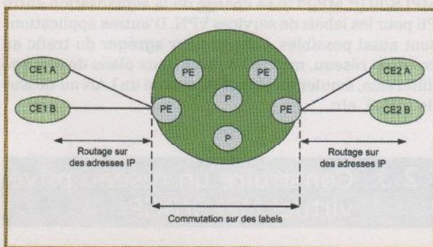
Figure 4 : Réseau implémentant des VPN MPLS/BGP
