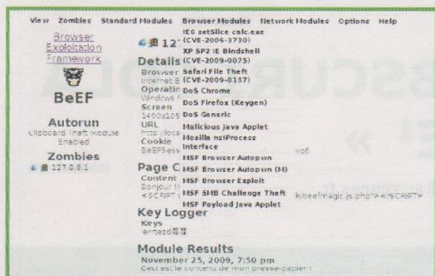
Fig. 2 : Le framework BeEF [43] permet de tester quelques-unes des possibilités offertes à un attaquant exploitant une vulnérabilité XSS pour prendre le contrôle d'un réseau de navigateurs zombies : visualisation du contenu de la page visitée, accès aux cookies de la page courante, keylogger, redirection, lancement d'exploits, notamment grâce à un interfaceage possible avec Metasploit 26 , etc.
