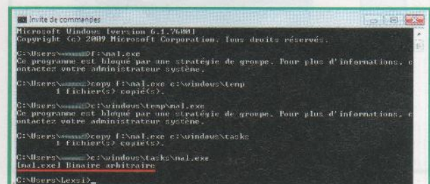
Contournement des règles AppLocker par défaut
