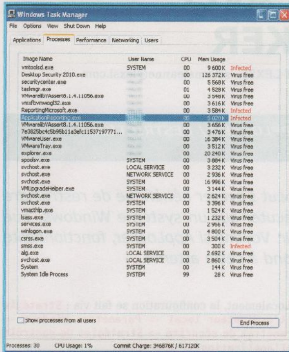
Fig. 7 : Gestionnaire des tâches après injection
