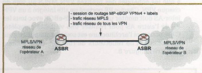
Figure 6 : Interconnexion - Option B
