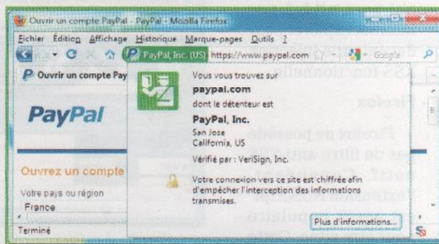
Fig. 2 : Affichage d'un certificat SSL EV dans Firefox
