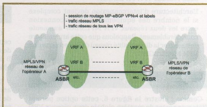
Figure 9 : Interconnexion - Option D (ou AB)
