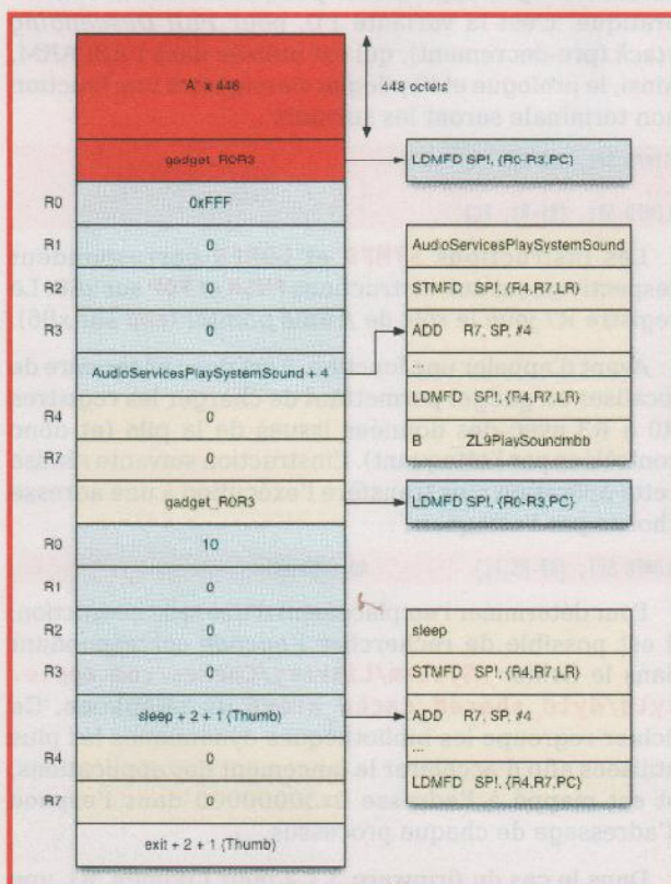
Figure 2 : Détail du payload
