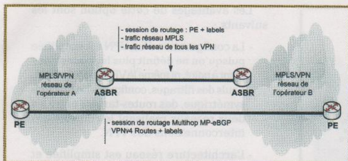
Figure 7 : Interconnexion - Option C avec session Multihop MP-eBGP entre les PE
