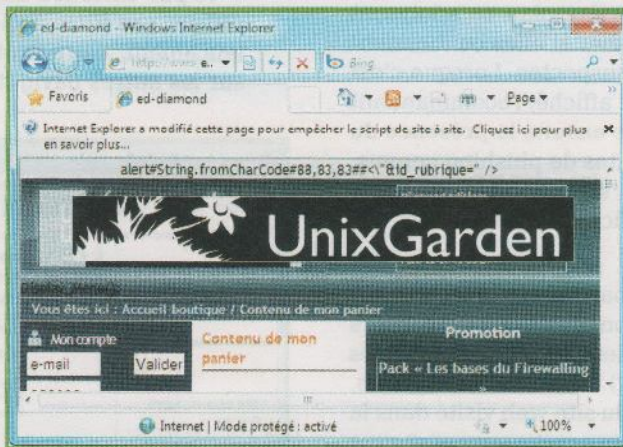
Fig. 3 : Le filtre anti-XSS d'Internet Explorer à l'œuvre
