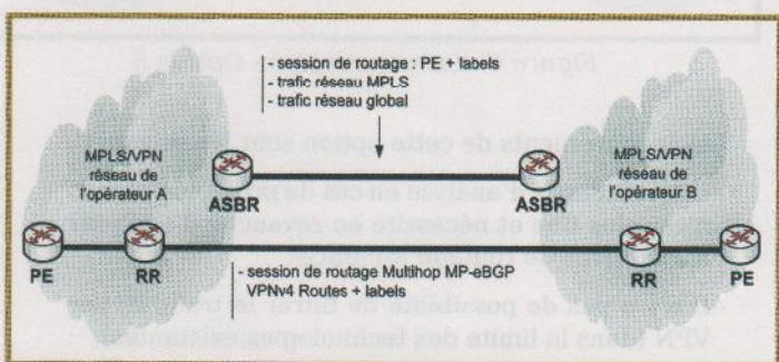
Figure 8 : Interconnexion - Option C avec session Multihop MP-eBGP entre les réflecteurs de routes
