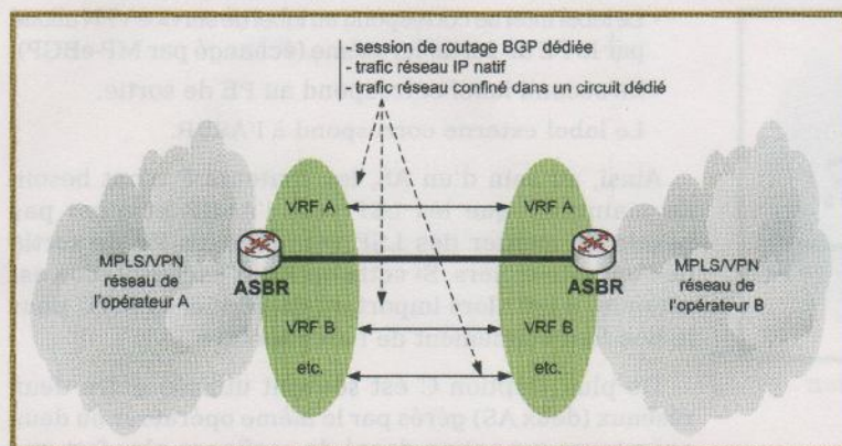
Figure 5 : Interconnexion - Option A
