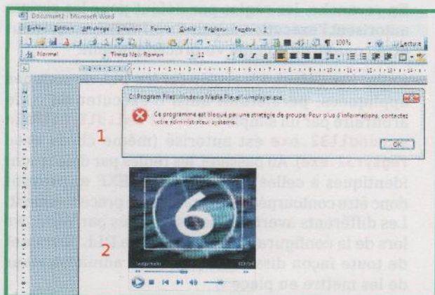
Contournement d'AppLocker via un contrôle ActiveX (Windows Media Player)
