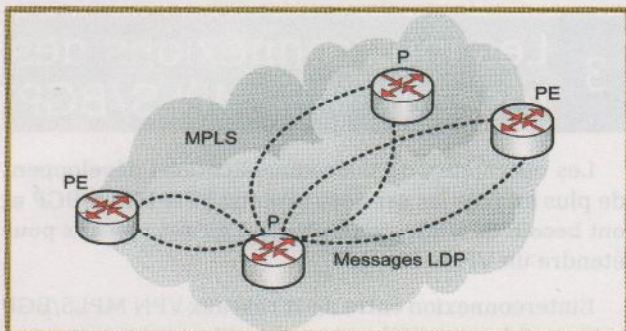
Figure 2 : Echange de messages LDP
