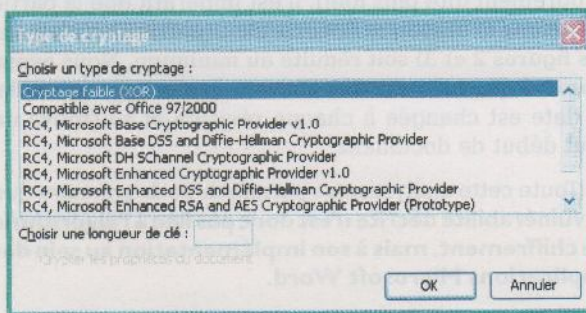
Figure 1 : Liste des chiffrements Word/Excel disponibles
